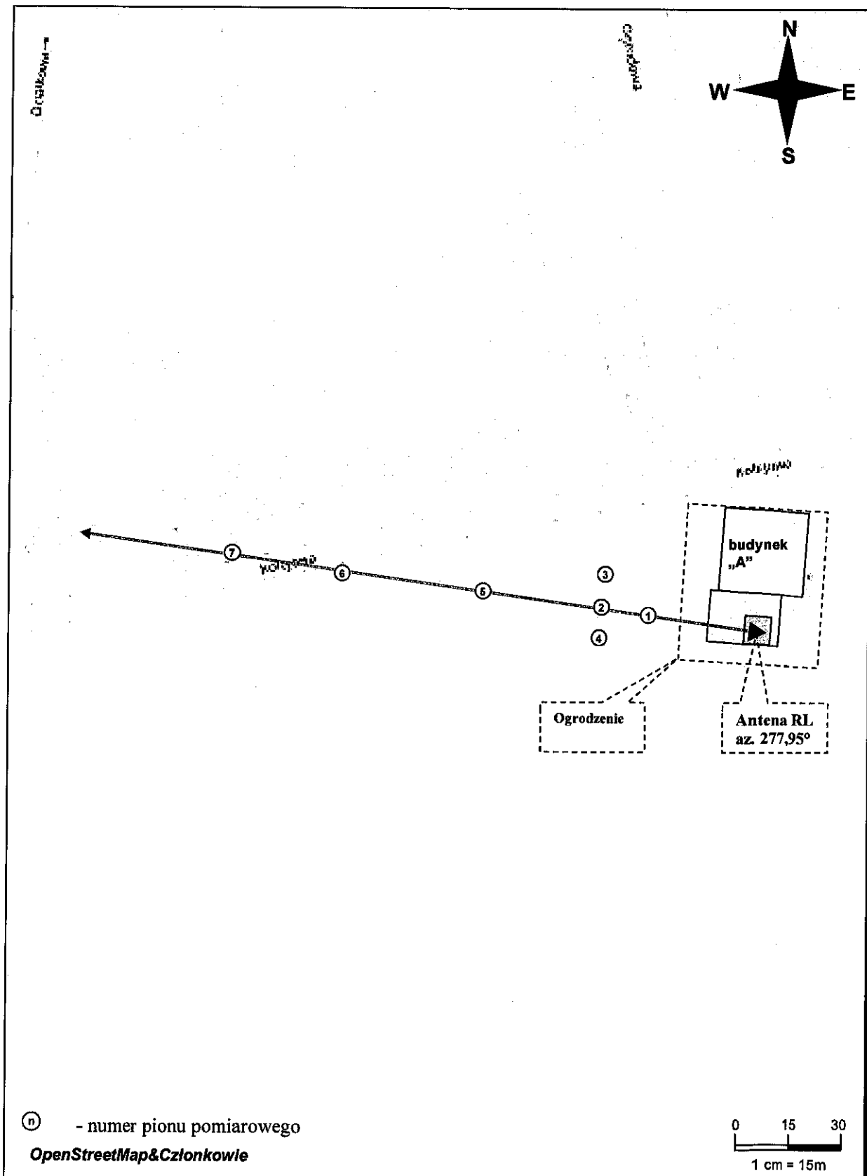
Rys. 1. Usytuowanie punktów i pionów pomiarowych w otoczeniu instalacji radiokomunikacyjnej Stacja Netia KOBZB147-KOBZM00038ANT001 Pustków Żurawski, ul. Kolejowa 13
